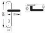
Mod. MONTAN mit Hochhaltefeder Drücker fest drehbar
