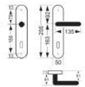
Mod. MARTHA ohne Hochhaltefeder
