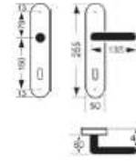
Mod. SELENE ohne Hochhaltefeder
